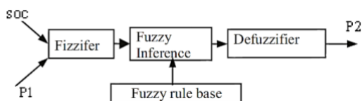
شکل ۱: ترکیب‌بندی پیشنهادی کنترل‌کننده فازی با ۳ ورودی از طریق استنتاج فازی
